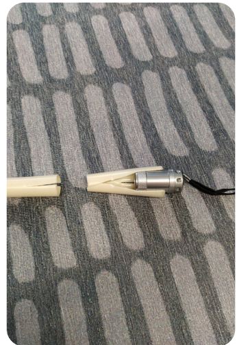
6. Tee kaksi halkeamaa myös teräosaan, jonka jälkeen voit ujuttaa kahvaosan n. 2cm teräosan sisään
